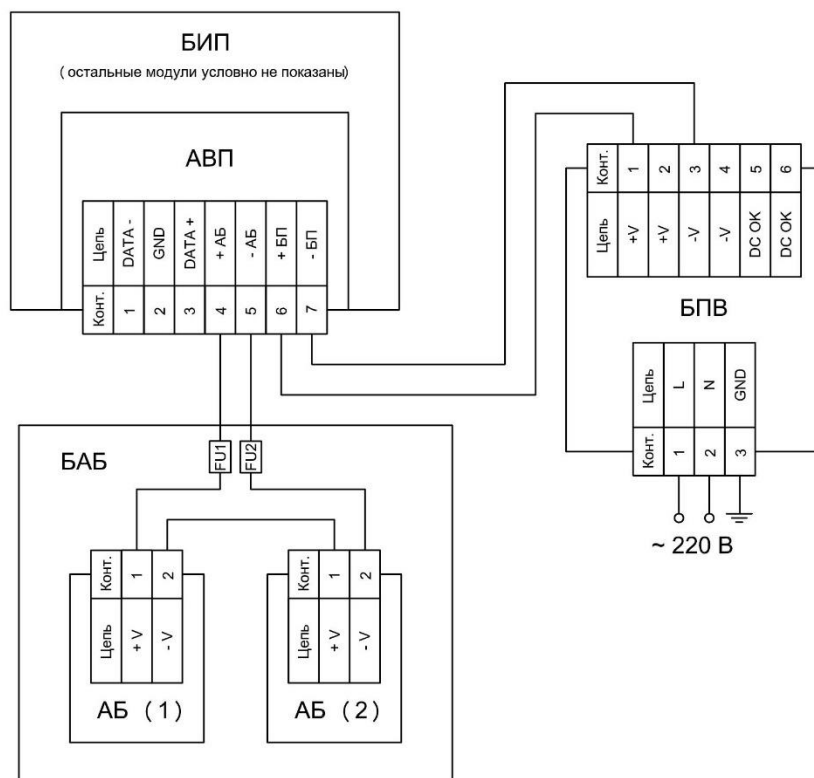
б) для БПВ марки MDR-60-24
