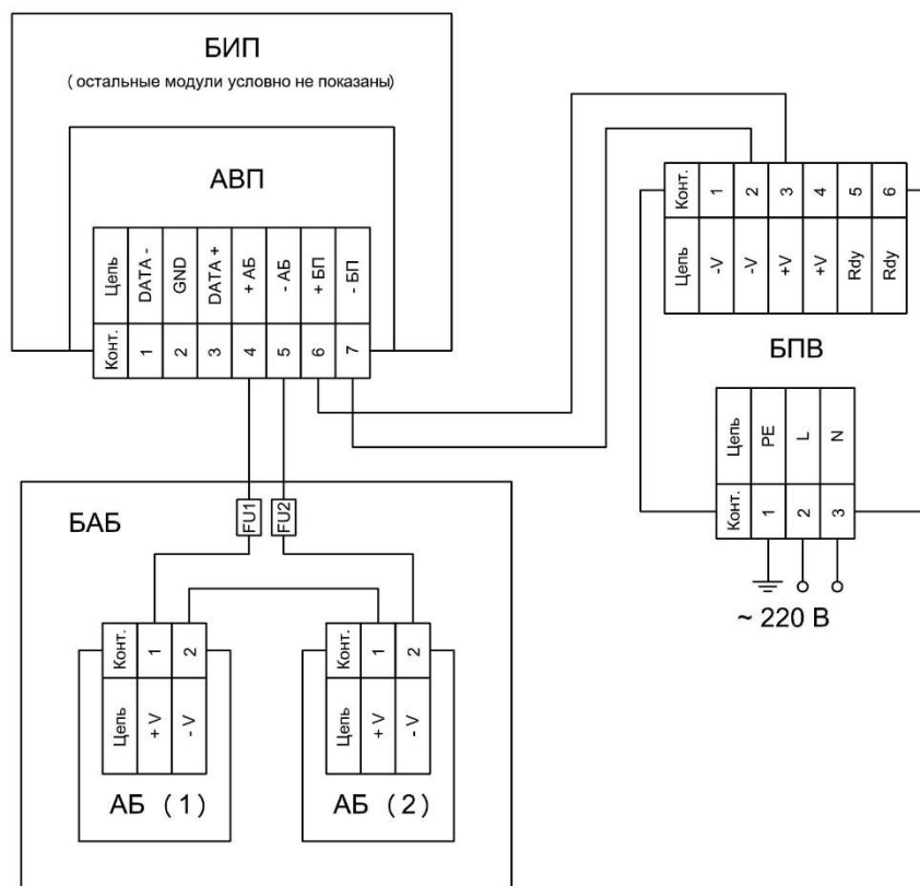
а) для БПВ марки NDR-75-24
