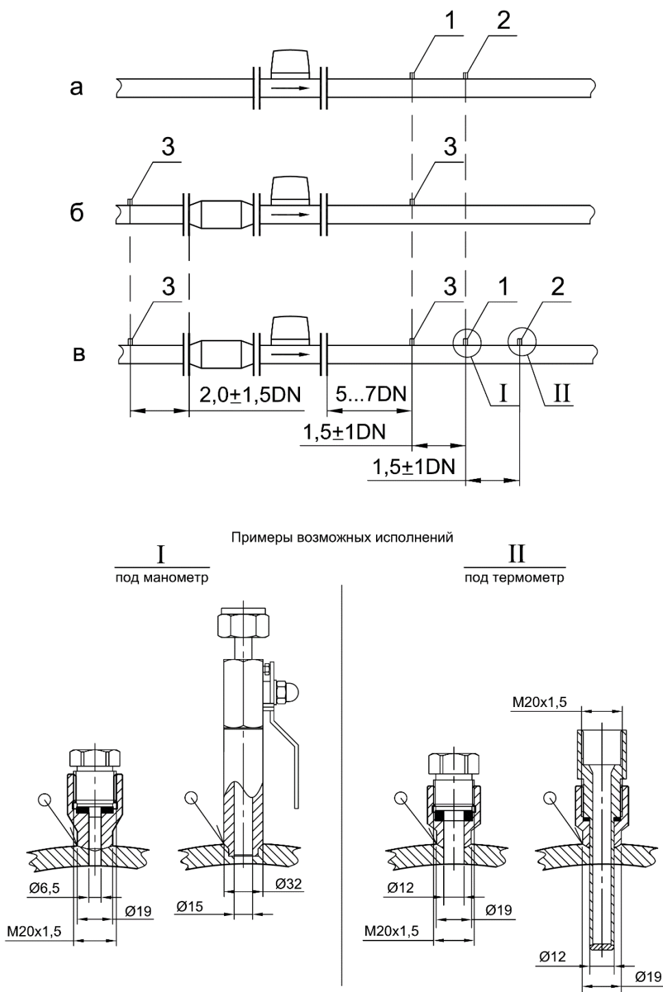
Рисунок Г.5 – «Врезка» штуцеров в ЭТ при монтаже ПП ИРВИС-Ультра-Пл
