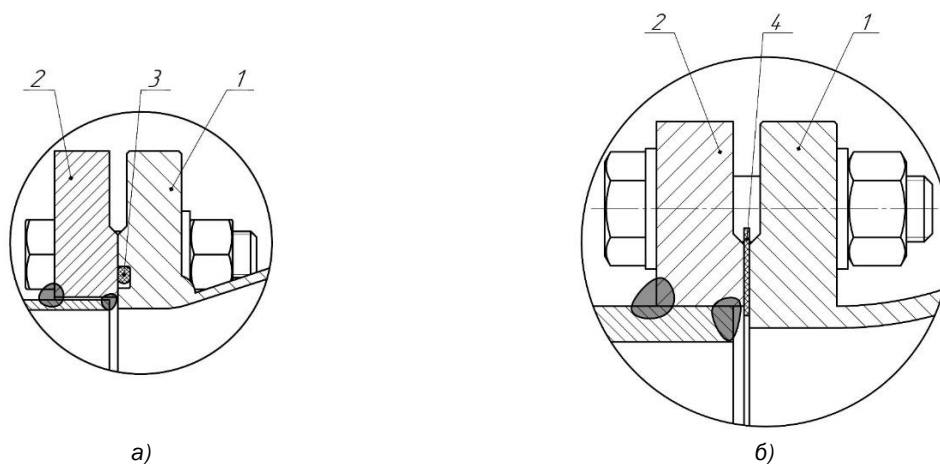
Рисунок Г.4.1 – Типы фланцевых уплотнений между УПП и ЭТ
