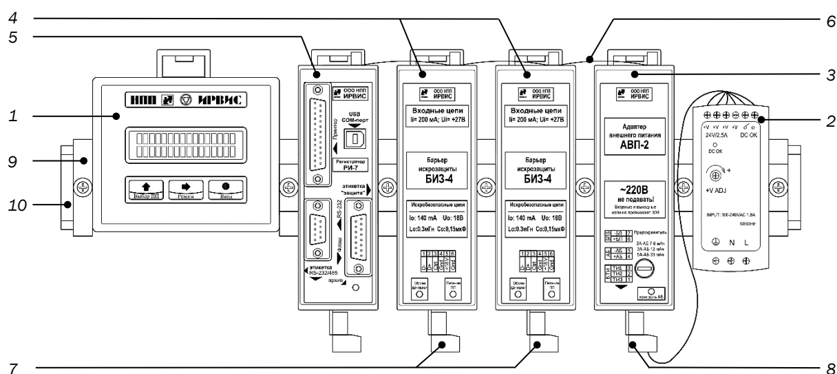
Рисунок 4 – Внешний вид БИП в бескорпусном исполнении (двухканальный вариант) 1 – БИ; 2 – БПС; 3 – АВП; 4 – БИЗ; 5 – РИ; 6 – КК; 7 – Вилка контактной системы для подключения СК; 8 – Вилка контактной системы для подключения кабеля питания 24 В и интерфейсного кабеля RS-485; 9 – Ограничитель; 10 – DIN-рейка
