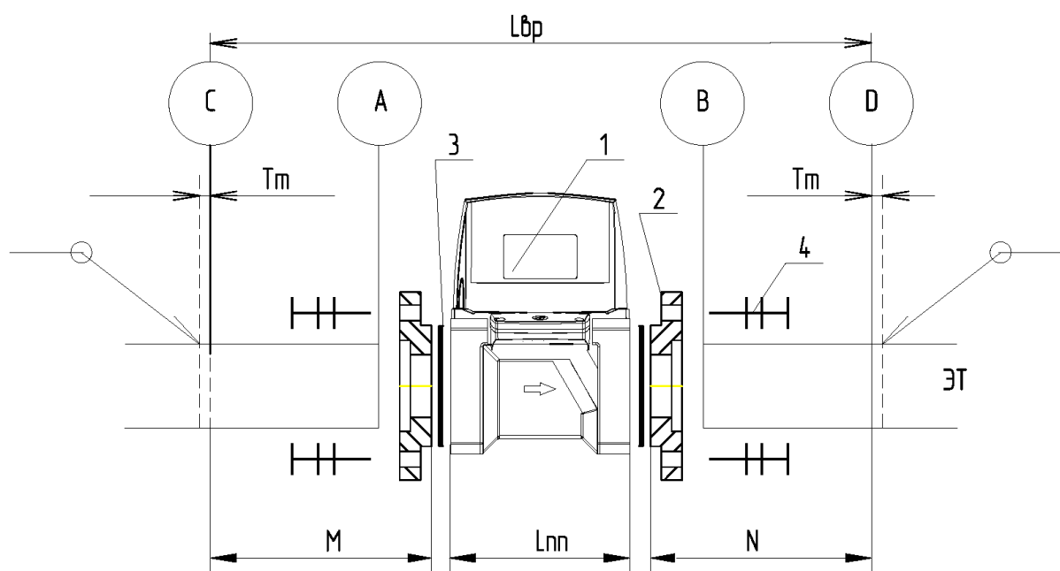
Рисунок Г.1 – Составные части участка «врезки» ИРВИС-Ультра-Пп-К 1 – ПП (имитатор ПП); 2 – Ответный фланец; 3 – Уплотнительная прокладка; 4 – Стандартный крепеж.
