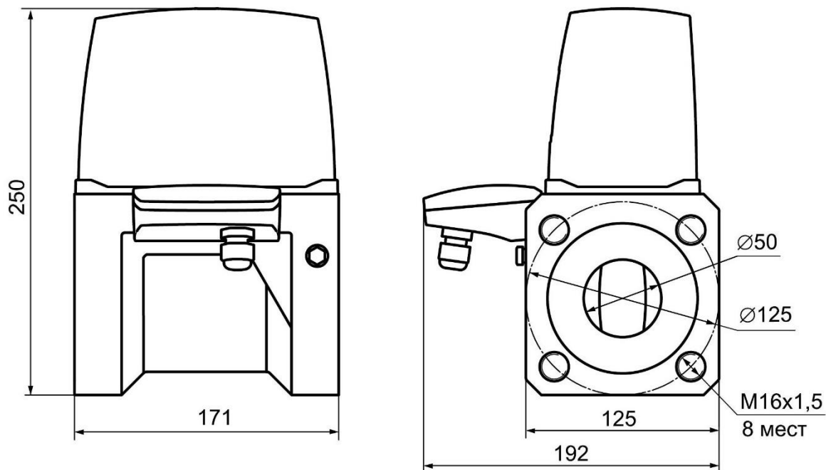
Рисунок Б.1 - Габаритные и присоединительные размеры ПП ИРВИС-Ультра-Пп-К-16-DN50
