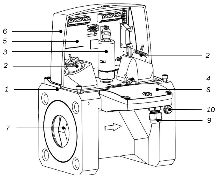
Рисунок 2 – Конструкция ПП ИРВИС-Ультра-Пп-К-16-DN50
