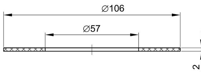
Рисунок Б.2 - Габаритные размеры уплотнительной прокладки ИРВИС-Ультра-Пп-К-16-DN50
