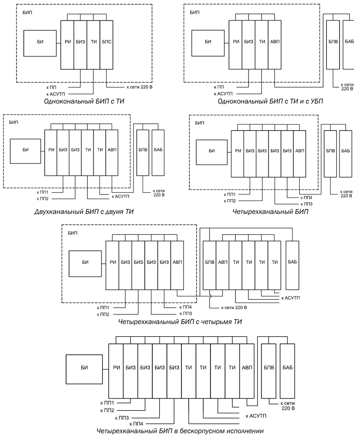
Рисунок Б.4 – Примеры вариантов исполнений БИП
